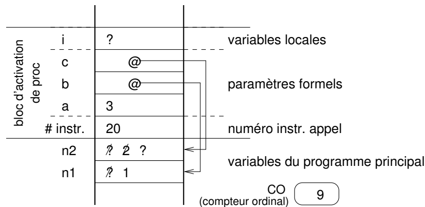
FIGURE 2 – État de la mémoire avant l'exécution du corps de la procédure
